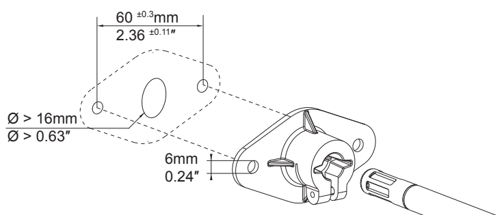
Abb. 7 Abmessungen Montageflansch
